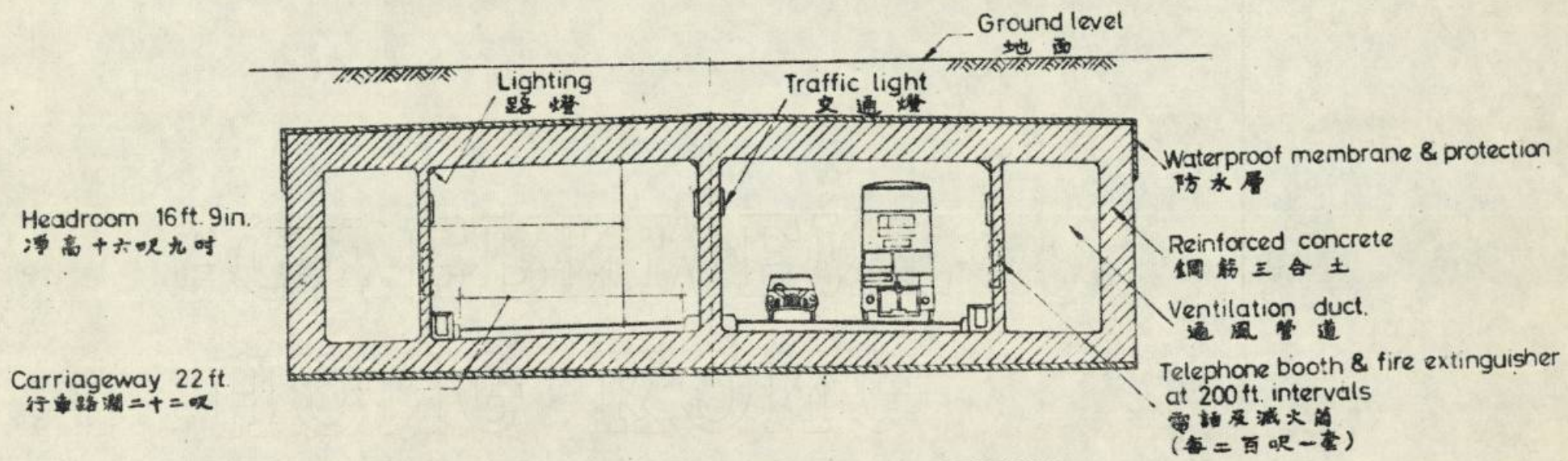
AIRPORT TUNNEL ROAD : CROSS-SECTION 機場行車隧道 : 橫切面
